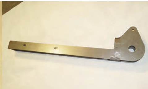
Hanger Wldmt. P/N P90.1067C (2x)
